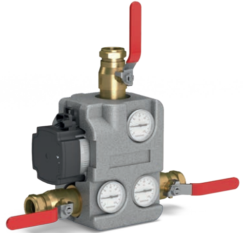
EPS-eristeellä / EPS isolering EPS insulation / EPS-Isolierung
